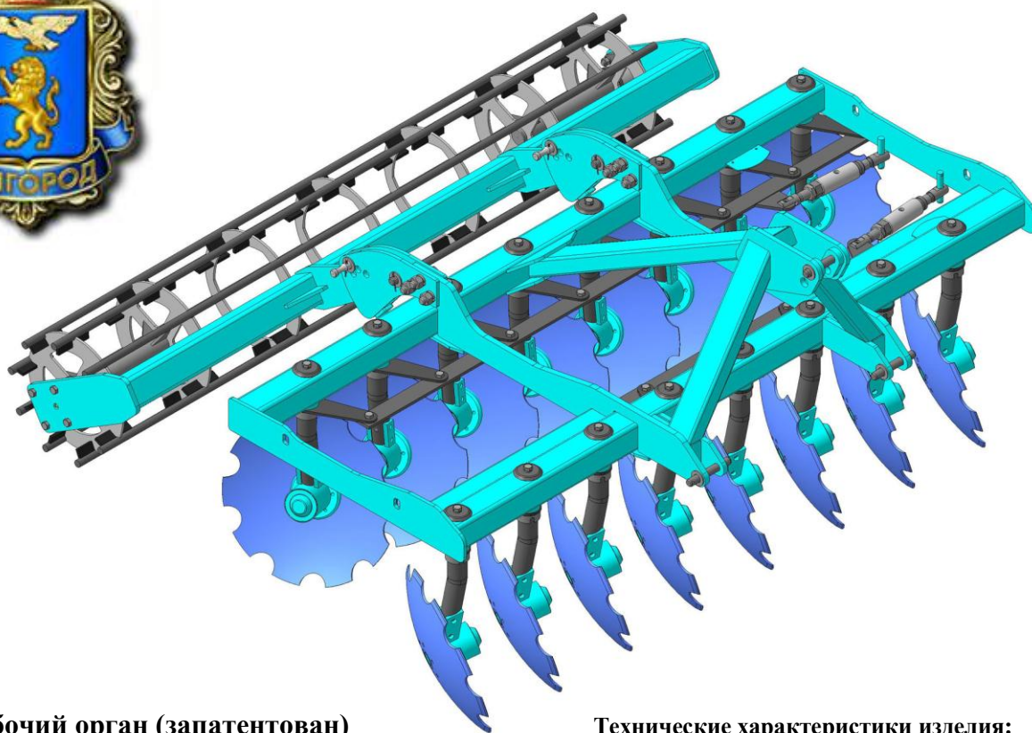
Рабочий орган (запатентован)
