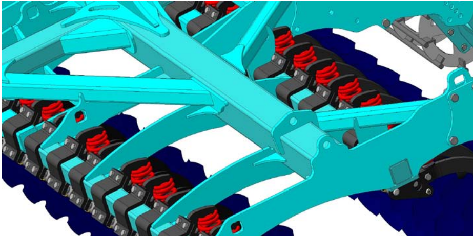
Мощное крепление снорца к раме.
